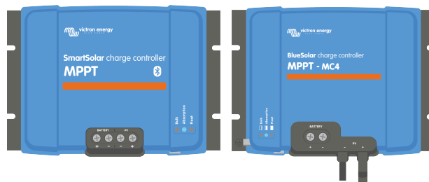
Von links nach rechts: Beispiel für Solarladegeräte mit Schraubklemmen und MC4-PV-Anschlüssen
