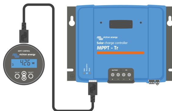
Verbinden Sie das Display mithilfe eines VE.Direct-Kabels mit dem Solarladegerät.
